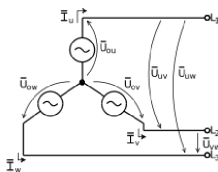
Zapojení do trojúhelníka
