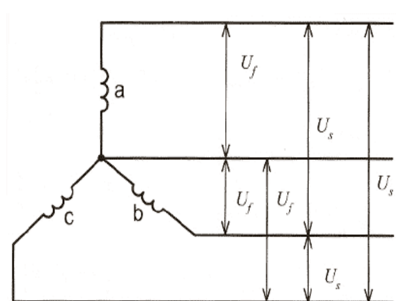
Zapojení do hvězdy
